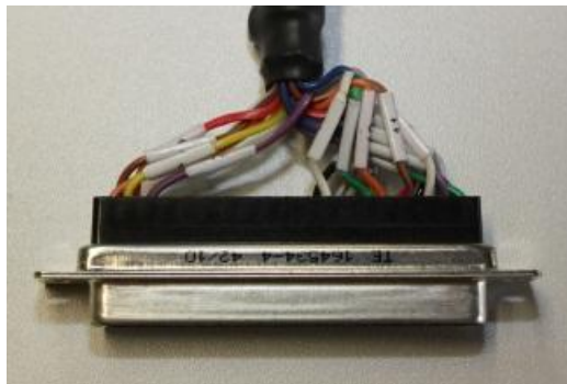
Konfektionierter Stecker
